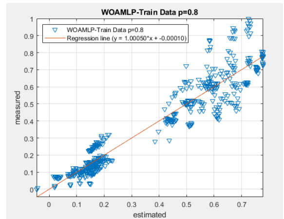
(d) WOAMLP train \alpha=0.8
